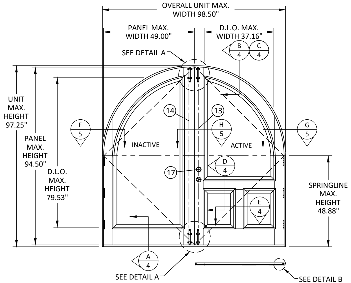
ELEVATION
